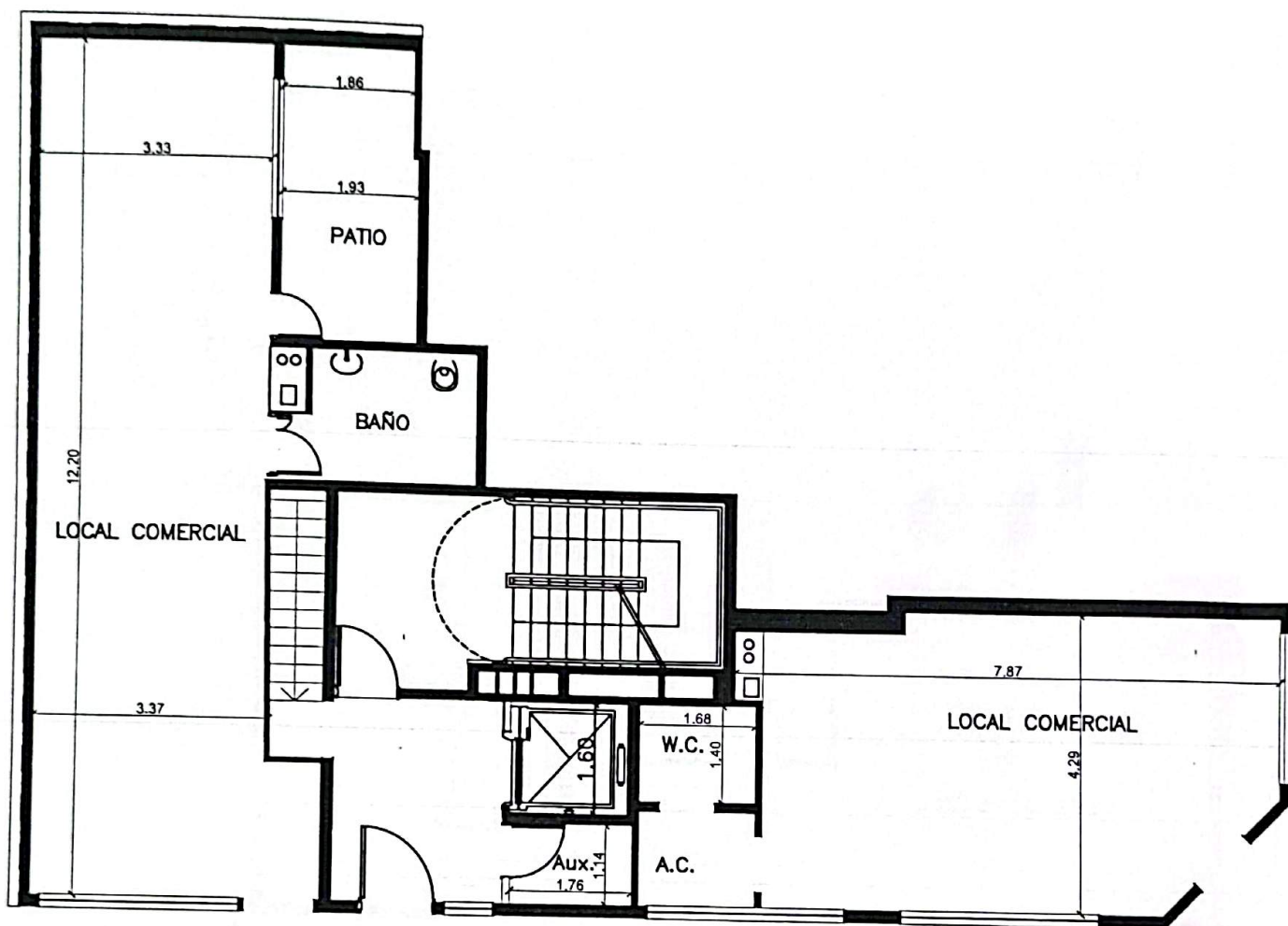
PLANTA BAJA 2
